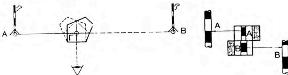
Σχ. 45 Διαδικασία πύκνωσης ευθυγραμμίας με το ορθόγωνο.
