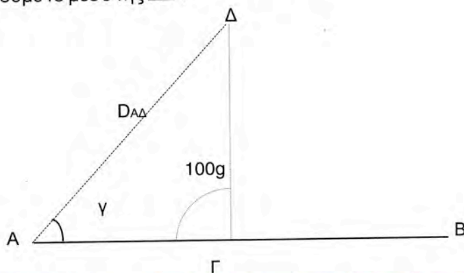
Σχ. 52 Χάραξη κάθετης σε ευθυγραμμία από σημείο Γ αυτής με θεοδόλιχο.
