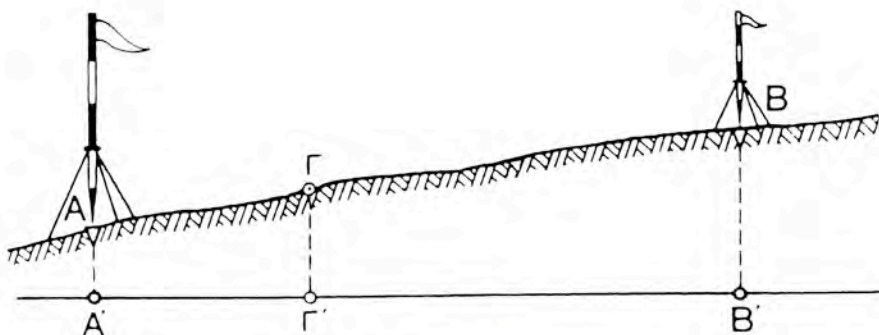
Σχ. 41 Οπτική πυκνωση ευθυγραμμίας.
