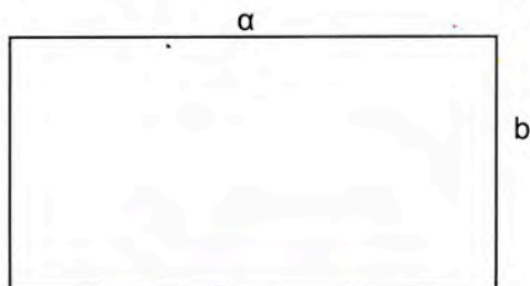
Σχ. 63 Ορθογώνιο
