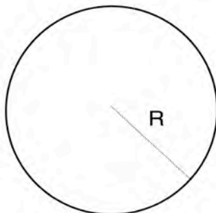
Σχ. 66 Κύκλος
