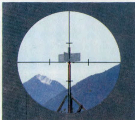
Εικ.11 Το σταυρόνημα όπως φαίνεται μέσα από το τηλεσκόπιο την ώρα της σκόπευσης.
