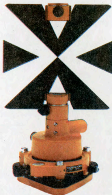
Εικ. 13 Ειδικός στόχος για μετρήσεις γωνιών.
