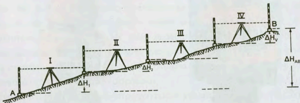
Σχ. 36 Εφαρμογή της χωροσταθμικής οδευσης.
