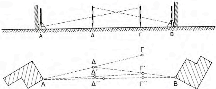
Σχ. 43 Τρόπος πύκνωσης ευθυγραμμίας όταν τα άκρα της είναι γωνίες κτιρίων.
