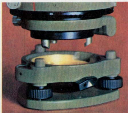
Εικ.9 Τρικόχλιο θεοδόλιχου.
