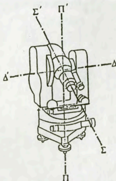
Σχ.20 Σχηματική παράσταση ενός θεοδολίχου με τους τρεις άξονές του.
