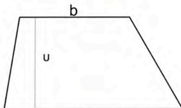
Σχ. 65 Τραπέζιο.
