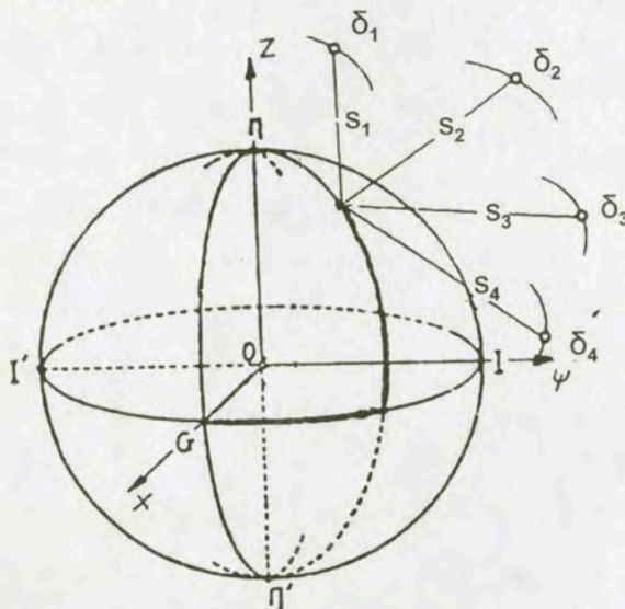
Σχ.17 Παρουσιάζεται η Γη με το παγκόσμιο τρισσορθόγωνιο σύστημα αναφοράς και οι δορυφόροι \delta_1, \delta_2, \delta_3, \delta_4 .
