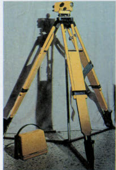
Χωροβάτης ευθύγραμμη σκοπευτικής γραμμής
