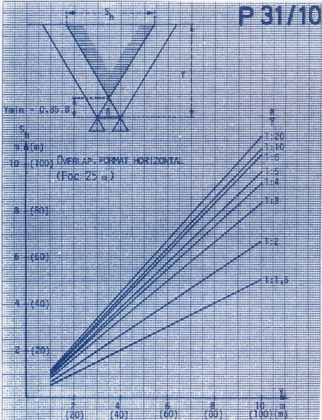
σχήμα 6.36 Νομογράφημα
