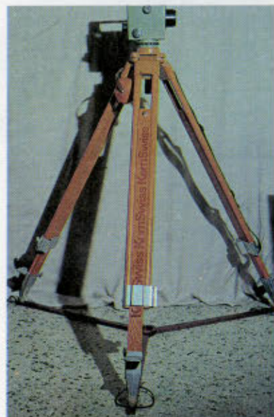
Χωροβάτης ευθύγραμμη σκοπευτικής γραμμής από δύο ορθογώνιες ανακλάσεις
