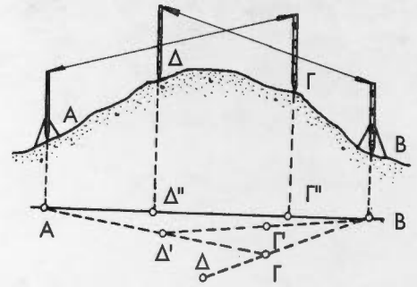
Πύκνωση ευθυγραμμίας μεταξύ δύο σημείων που είναι αμοιβαία ορατά
