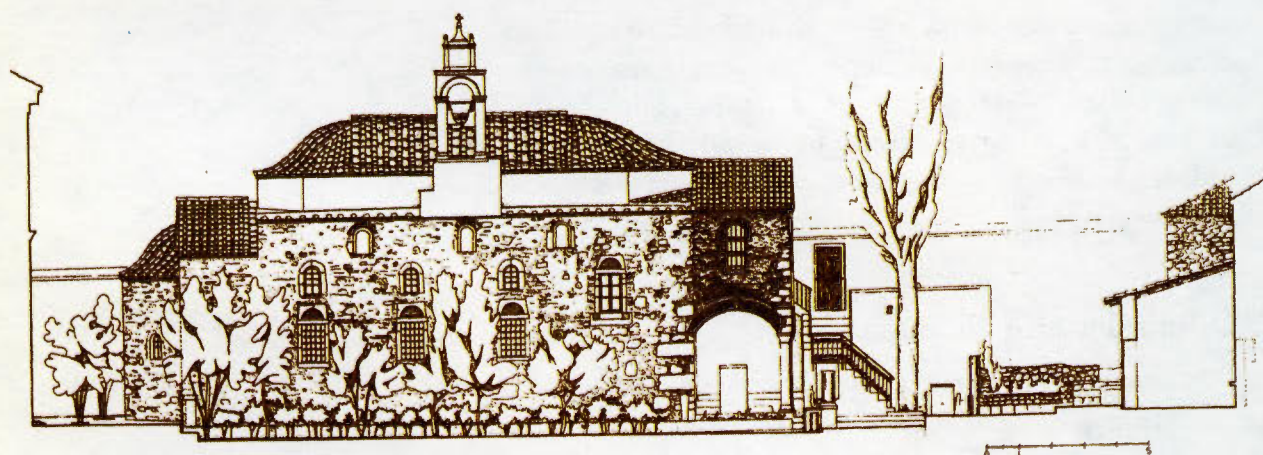
Μετόχι Παναγίου Τάφου, Πλάκα. Τομή - Όψη (Αποτύπωση Α. Πορτελάνος)
