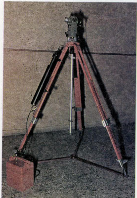
Θεοδόλιχο εφοδιασμένο με συσκευή laser
