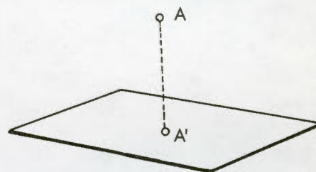
Ορθή προβολή σημείου σε επίπεδο
