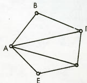
Επιμερισμός σχήματος σε τρίγωνα
