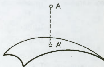
Ορθή προβολή σημείου σε επιφάνεια με καμπυλότητα
