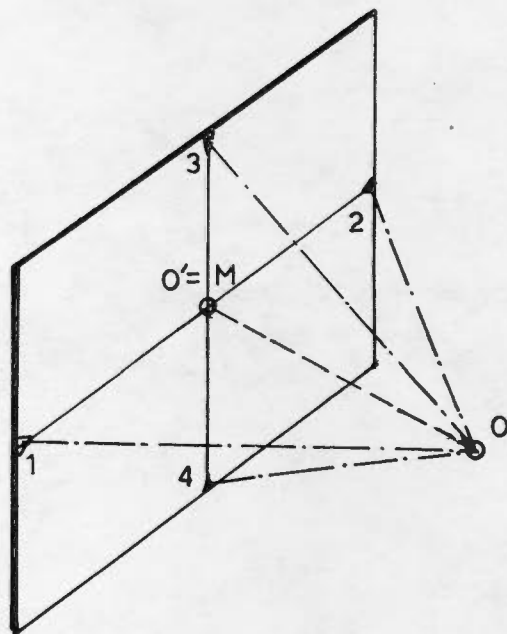
σχήμα 6.3 Εσωτερικός προσανατολισμός μετρητικών φωτομηχανών
