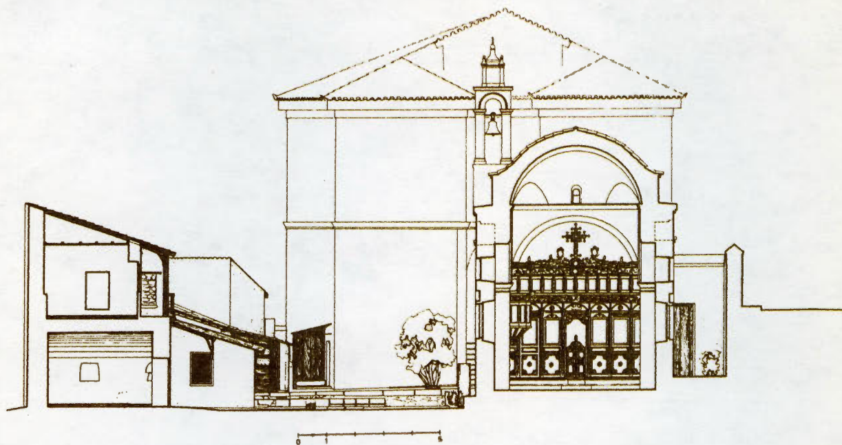
Μετόχι Παναγίου Τάφου, Πλάκα. Τομή - Όψη (Αποτύπωση Α. Πορτελάνος)
