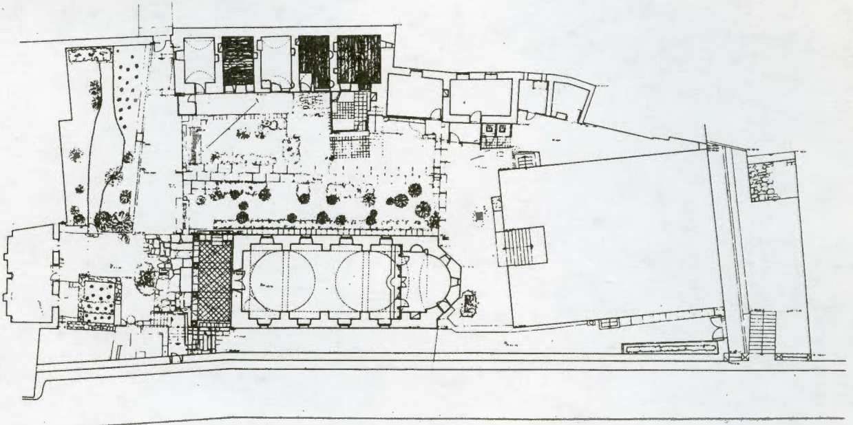
Μετόχι Παναγίου Τάφου. - Πλάκα - Κάτοψη συγκροτήματος Β' στάθμη
