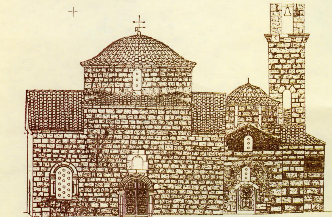
Άγιοι Απόστολοι Καλαμάτας. Πρόταση αποκατάστασης. Νότια όψη. (Α. Πορτελάνος)
