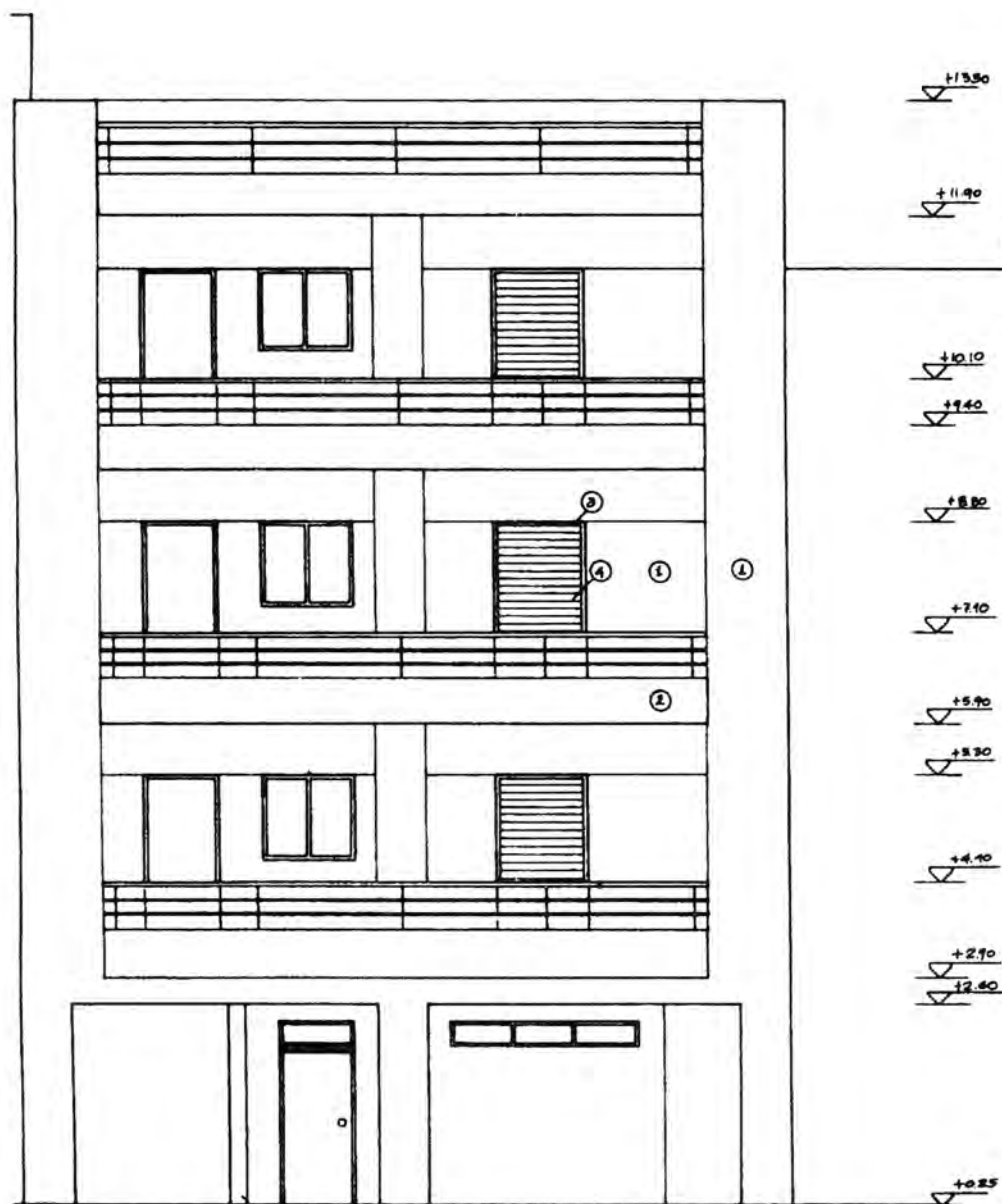
Εικ. 121 Όψη πολυώροφης κατοικίας.
